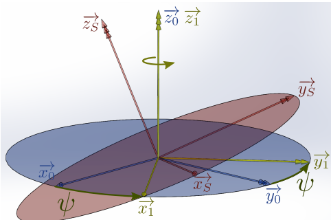
(a) Angle de précession \psi = (\vec{x}_0, \vec{x}_1) = (\vec{y}_0, \vec{y}_1)
