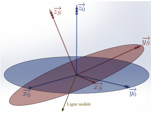
FIG. 7 – Construction de la ligne nodale
