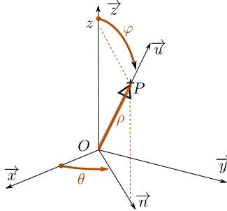
FIG. 4 – Repère sphérique
