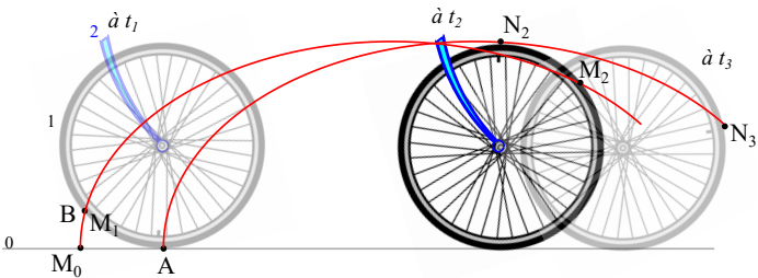
FIG. 1 – Points coïncidents à une date t
