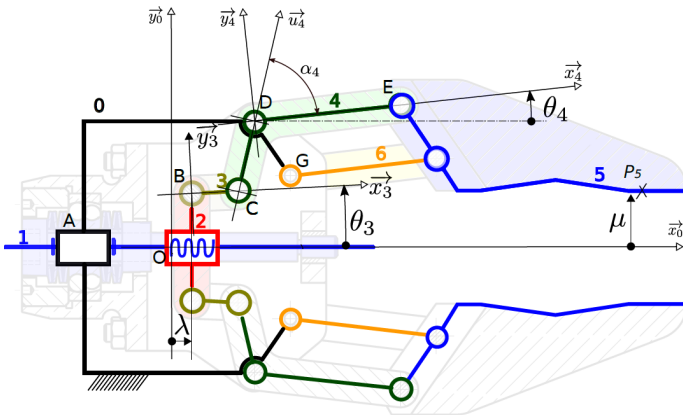
FIG. 5 – Combinaison de repères
