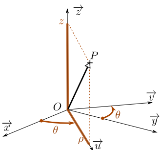
FIG. 3 – Repère cylindrique
